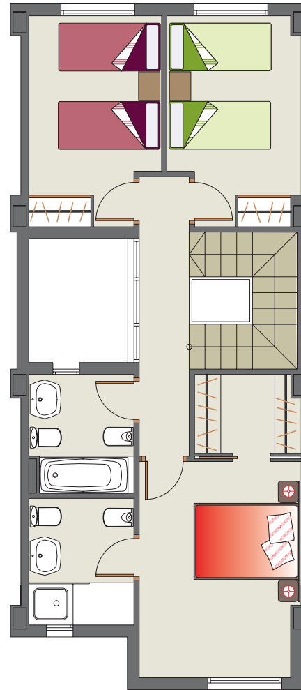
PLANTA SEGUNDA
